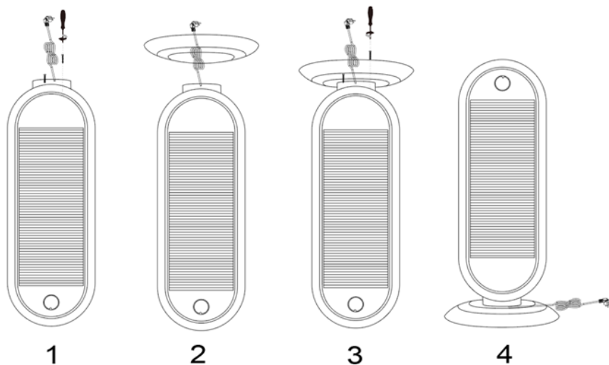
Рис.2 Установка/снятие опоры
